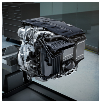
Động cơ 2.0L mới với công nghệ 48V mild-hybrid được lắp ráp theo triết lý "ONE MAN, ONE ENGINE"
